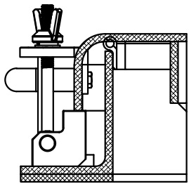
kveTi A-A
