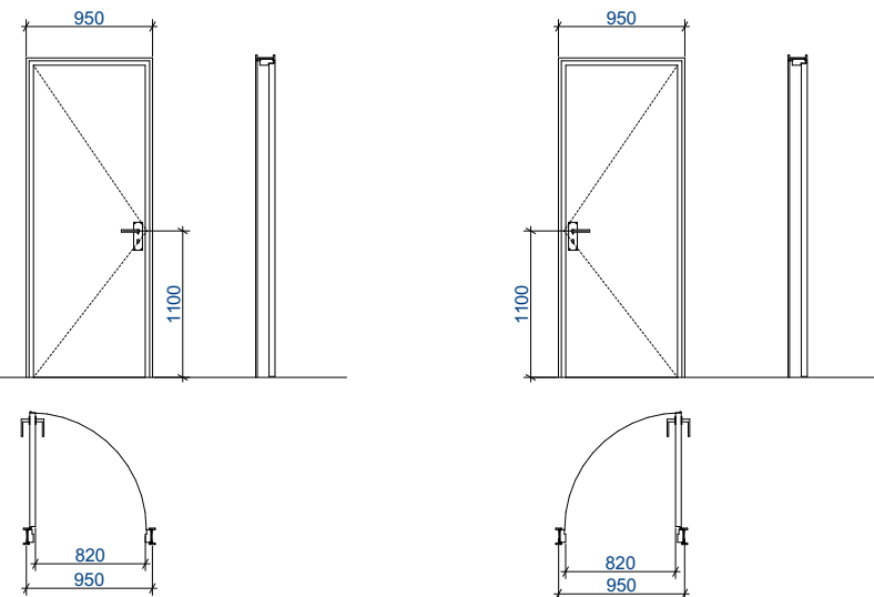
კ-3 კარი ზღურბლის და მიმხურავის გარეშე
