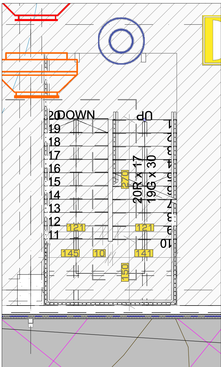
კიბის უპრადი #2 +6,90 ნიშნულზე 1:50
