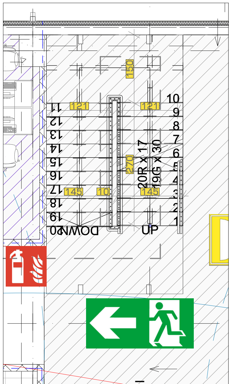
კიბის უპრადი #1 +0,00 ნიშნულზე 1:50
