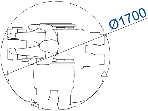
მოსატრიალებელი სივრცეები ვარიანტი 4
