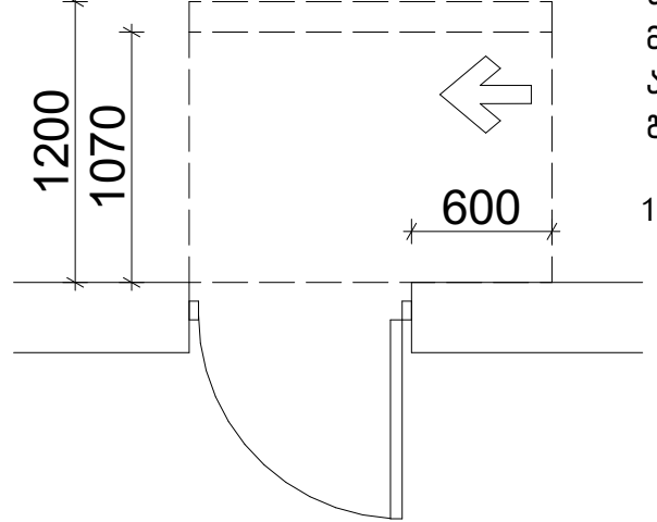
თავისუფალი სივრცე კართან მანევრირებისთვის - ანჟამიანი კარი ანჟამის მხრიდან მისაწვდომი - მიწოლით გაღება 120 მიწ. თუ მოწყობილია მიმხურავი
