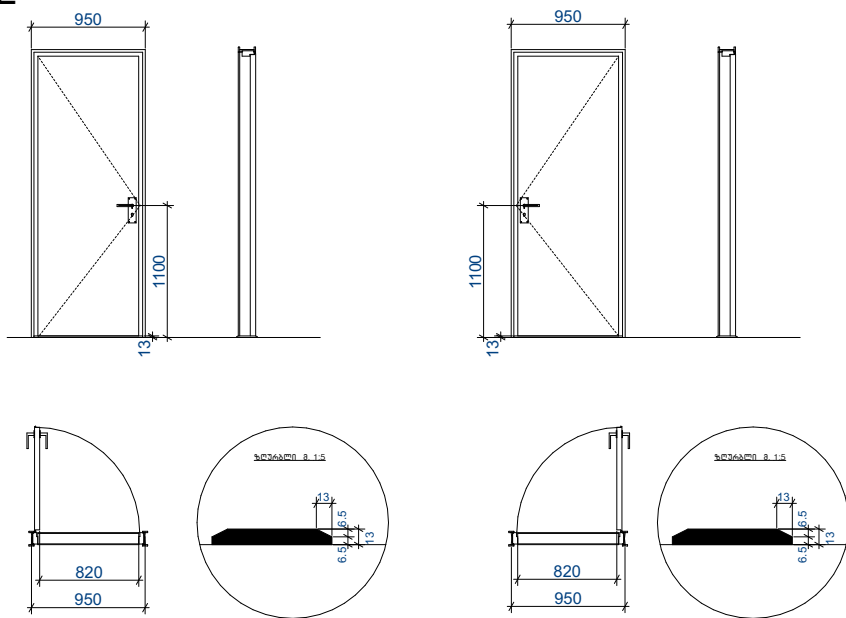
კ-2 კარი ზღურბლით მიმხურავის გარეშე
