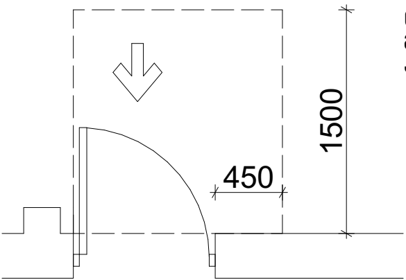
თავისუფალი სივრცე კართან მანევრირებისთვის-წინაგზი მოწყობილი კარი და ჭიშკარი-გამონებით გაღება
