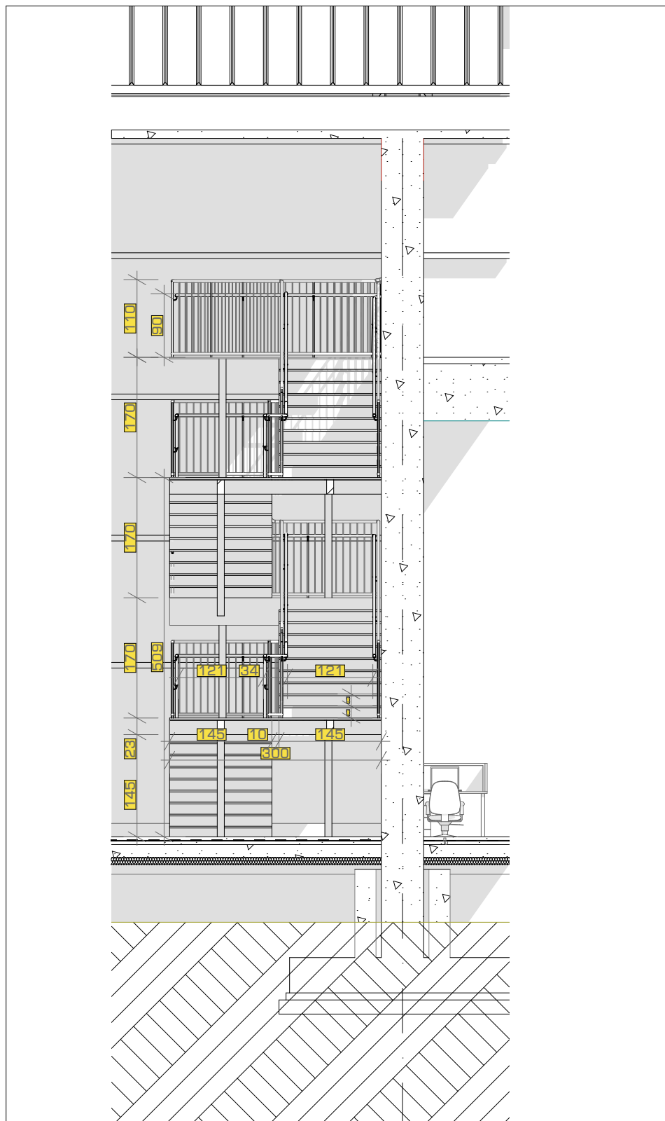
მოპირის დეტალი 1:75
