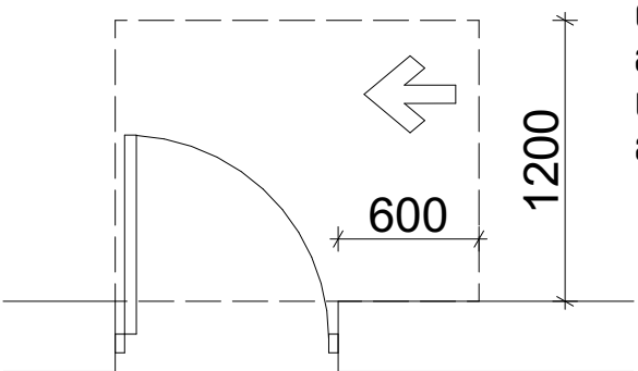
თავისუფალი სივრცე კართან მანევრირებისთვის - ანჟამიანი კარი საქების მხრიდან მისაწვდომი - გამონებით გაღება
