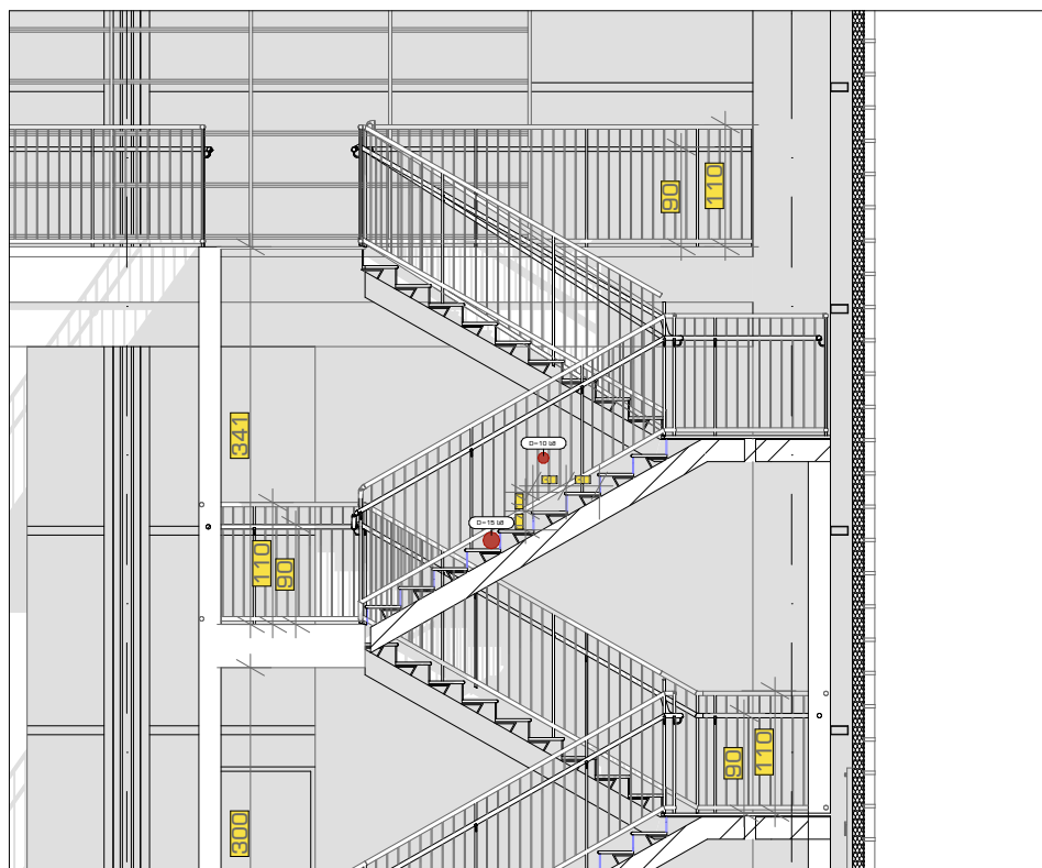
მოპირის დეტალი 1:75
