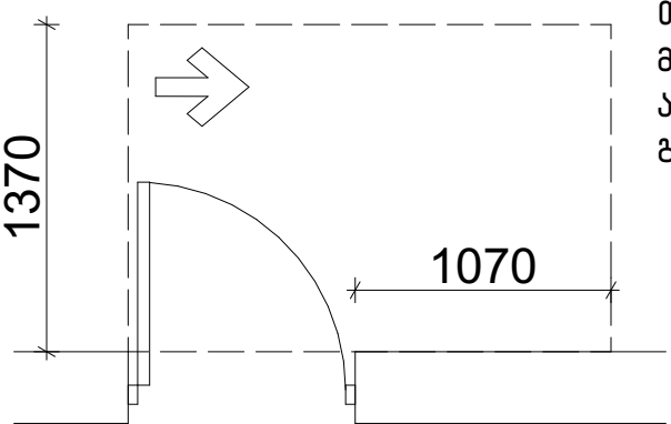
თავისუფალი სივრცე კართან მანევრირებისთვის - ანჟამიანი კარი ანჟამის მხრიდან მისაწვდომი - გამონებით გაღება
