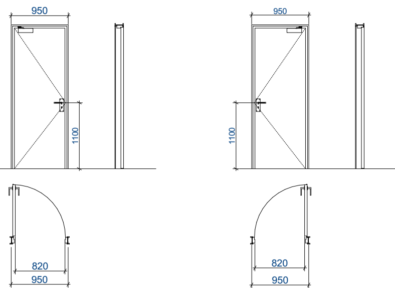
კ-1 კარი ზღურბლის გარეშე მიმხურავით
