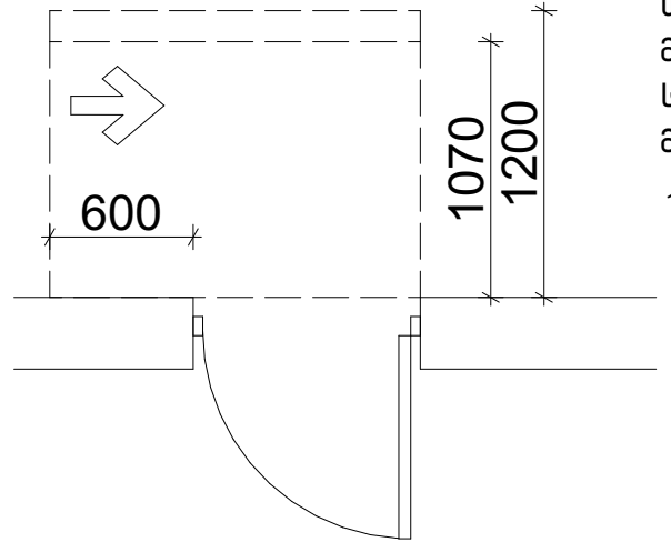
თავისუფალი სივრცე კართან მანევრირებისთვის - ანჟამიანი კარი საქების მხრიდან მისაწვდომი - მიწოლით გაღება 120 მიწ. თუ მოწყობილია მიმხურავი
