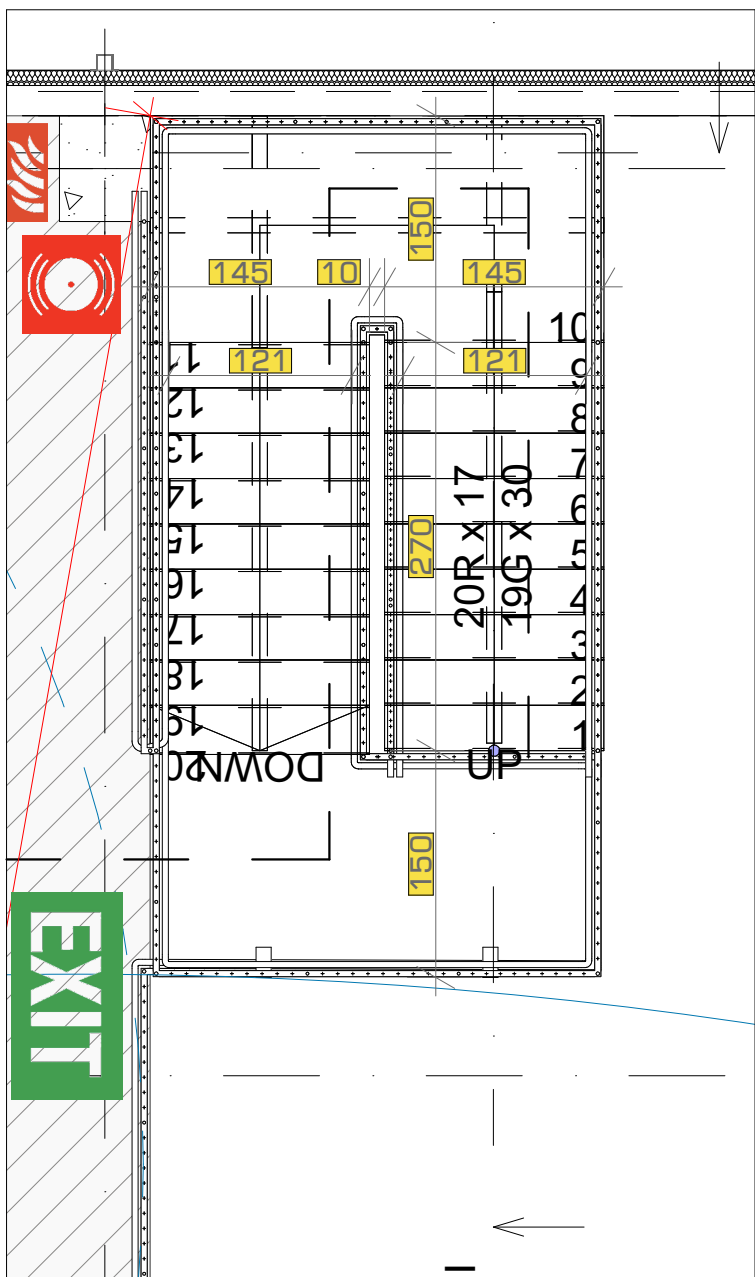
1. კიბის უპრადი #1 +6,90 ნიშნულზე 1:50
