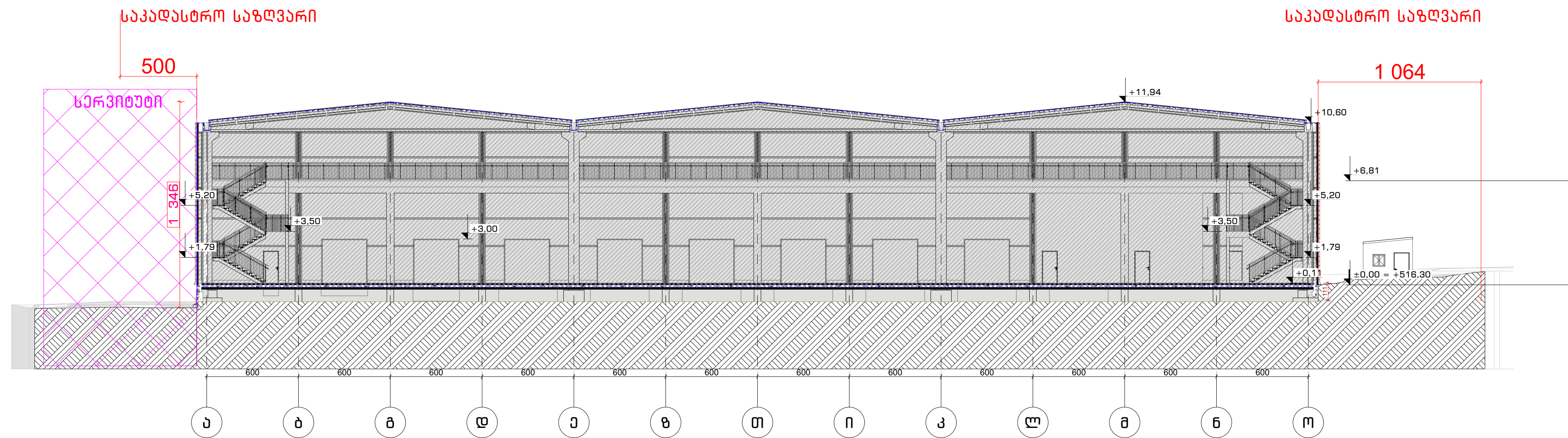
ჭრილი 1-1
