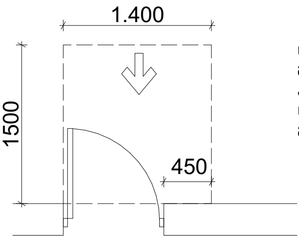
თავისუფალი სივრცე კართან მანევრირებისთვის - ანჟამიანი კარი წინიდან მისაწვდომი - გამონებით გაღება
