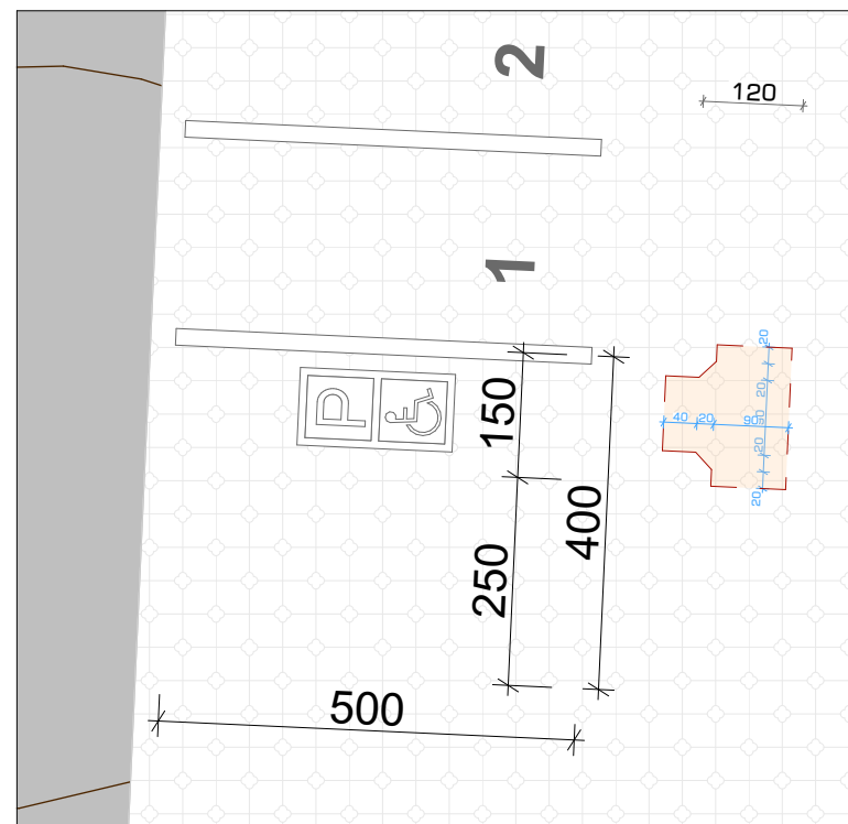
შშმ-ის პარკინგი 1:100
