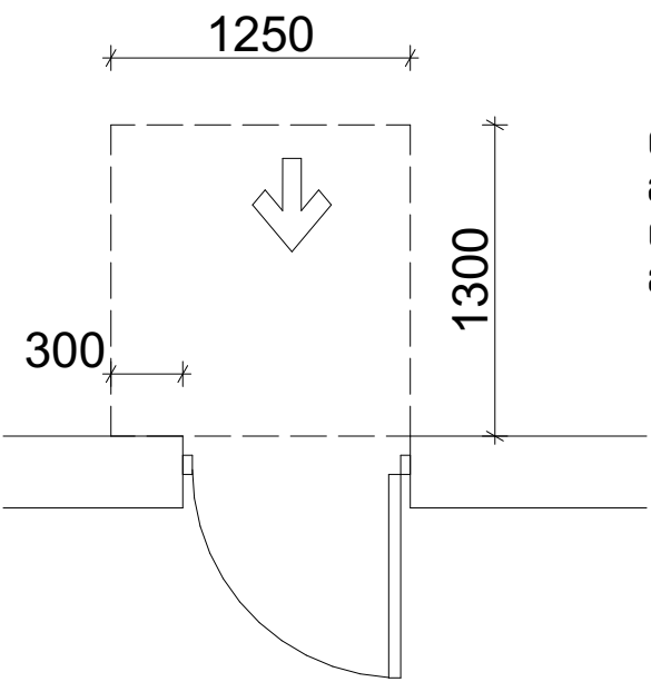
თავისუფალი სივრცე კართან მანევრირებისთვის - ანჟამიანი კარი წინიდან მისაწვდომი - მიწოლით გაღება
