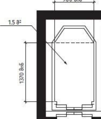
სურ. 407.4.1 (დ) კაბინის ბაბარტიბები - კარის ნიშნისმიერი მდებარეობა
