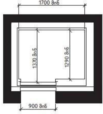
სურ. 407.4.1 (ა) კაბინის ბაბარტიბები - მინიმალური მდებარეობა კარში (მინიმალური მდებარეობა კარში)
