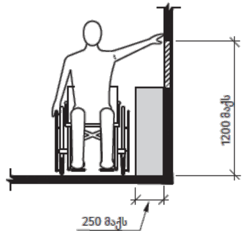
სურ. 308.3.2 (ბ) შეზღუდული მისაწვდომი
