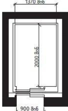
სურ. 407.4.1 (ბ) კაბინის ბაბარტიბები - კარის ნიშნისმიერი მდებარეობა
