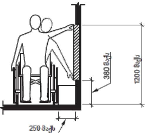
სურ. 308.3.1 შეზღუდული მისაწვდომი
