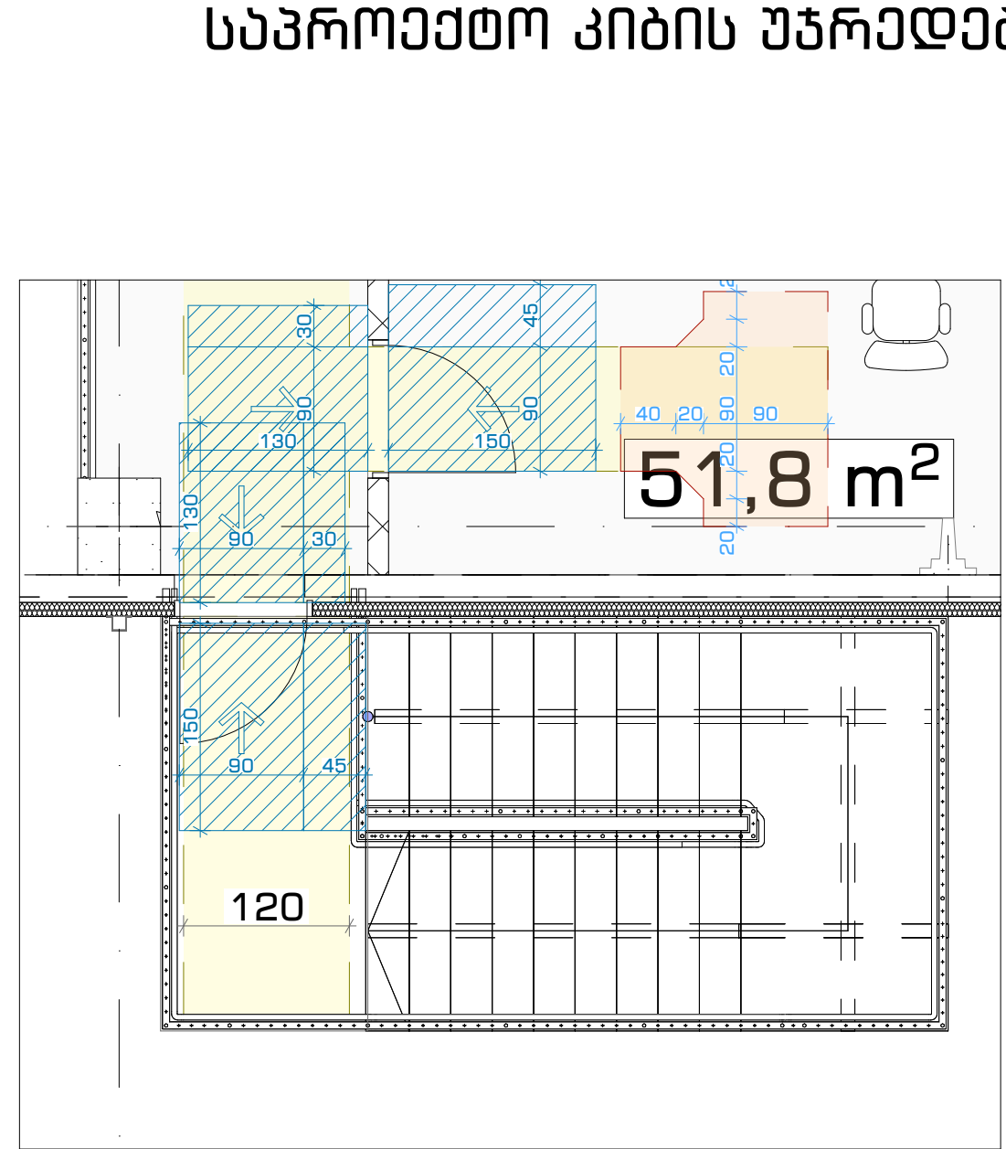
კიბის უბრედი +6,90 ნიშნულზე 1:50
