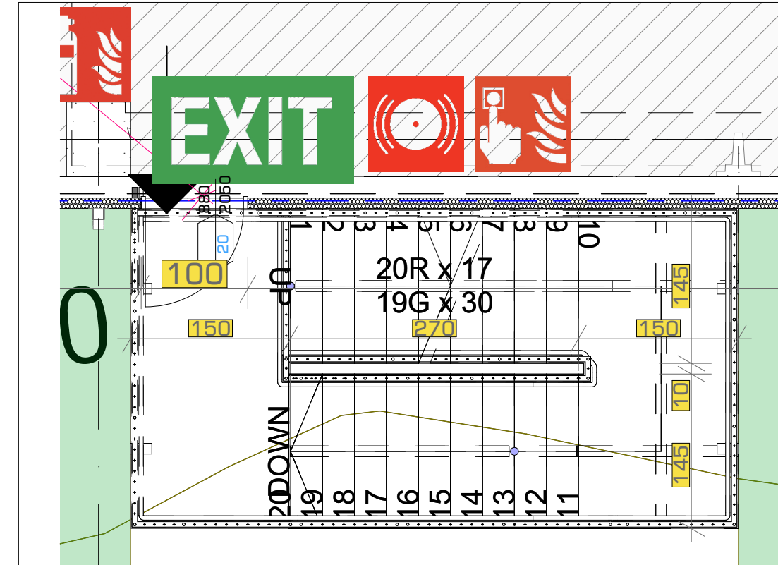
სახანძრო კიბის უბრედი +0,00 ნიშნულზე 1:50
