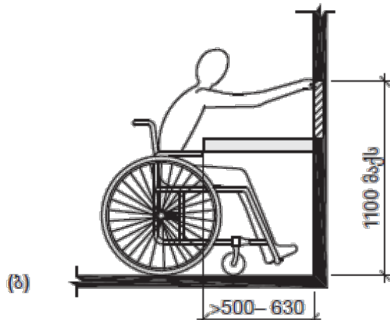
სურ. 308.2.2 შეზღუდული მისაწვდომი
