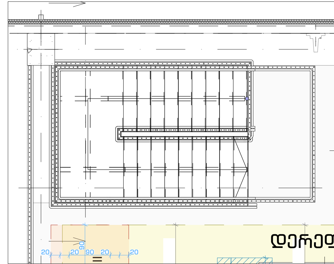
კიბის უბრედი +6,90 ნიშნულზე 1:50
