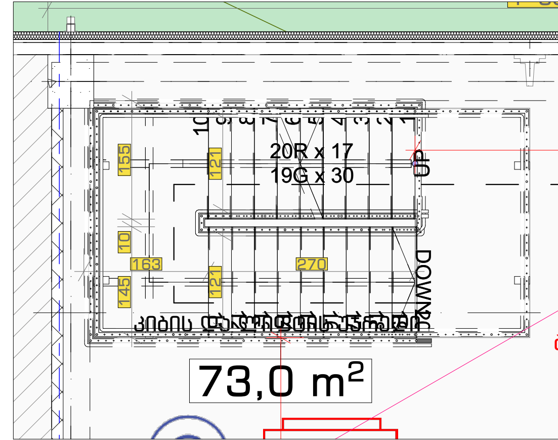
კიბის უბრედი +0,00 ნიშნულზე 1:50
