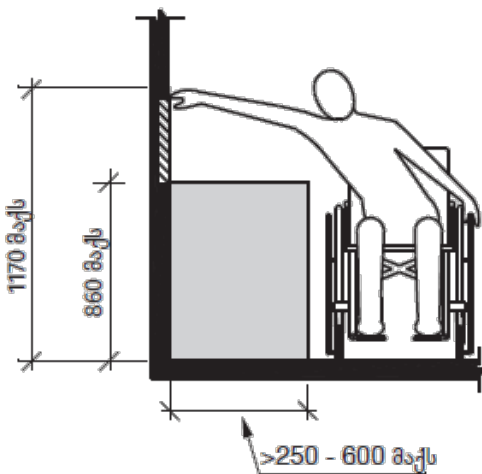
სურ. 308.3.2 (ბ) შეზღუდული მისაწვდომი
