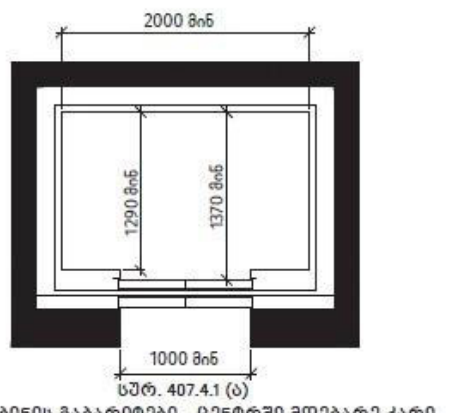
კაბინის ბაბარტიბები - მინიმალური მდებარეობა კარში
