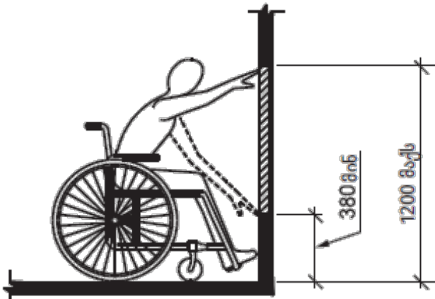
სურ. 308.2.1 შეზღუდული მისაწვდომი
