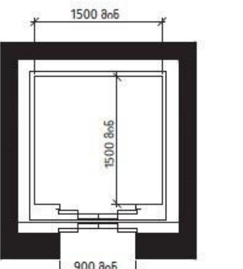
სურ. 407.4.1 (გ) კაბინის ბაბარტიბები - კარის ნიშნისმიერი მდებარეობა
