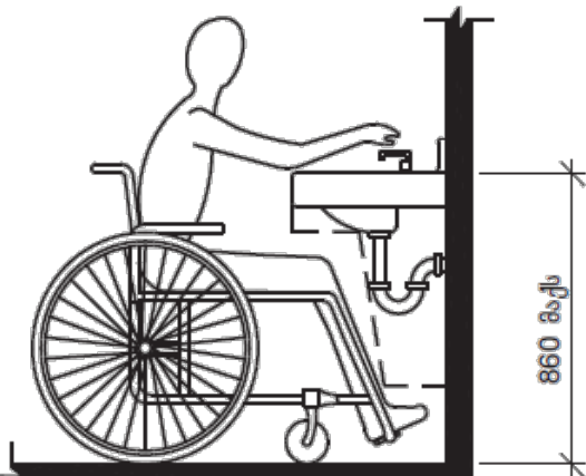
სურათი 606.3 ხელსაბბნების და ნიშნების სიმაღლე
