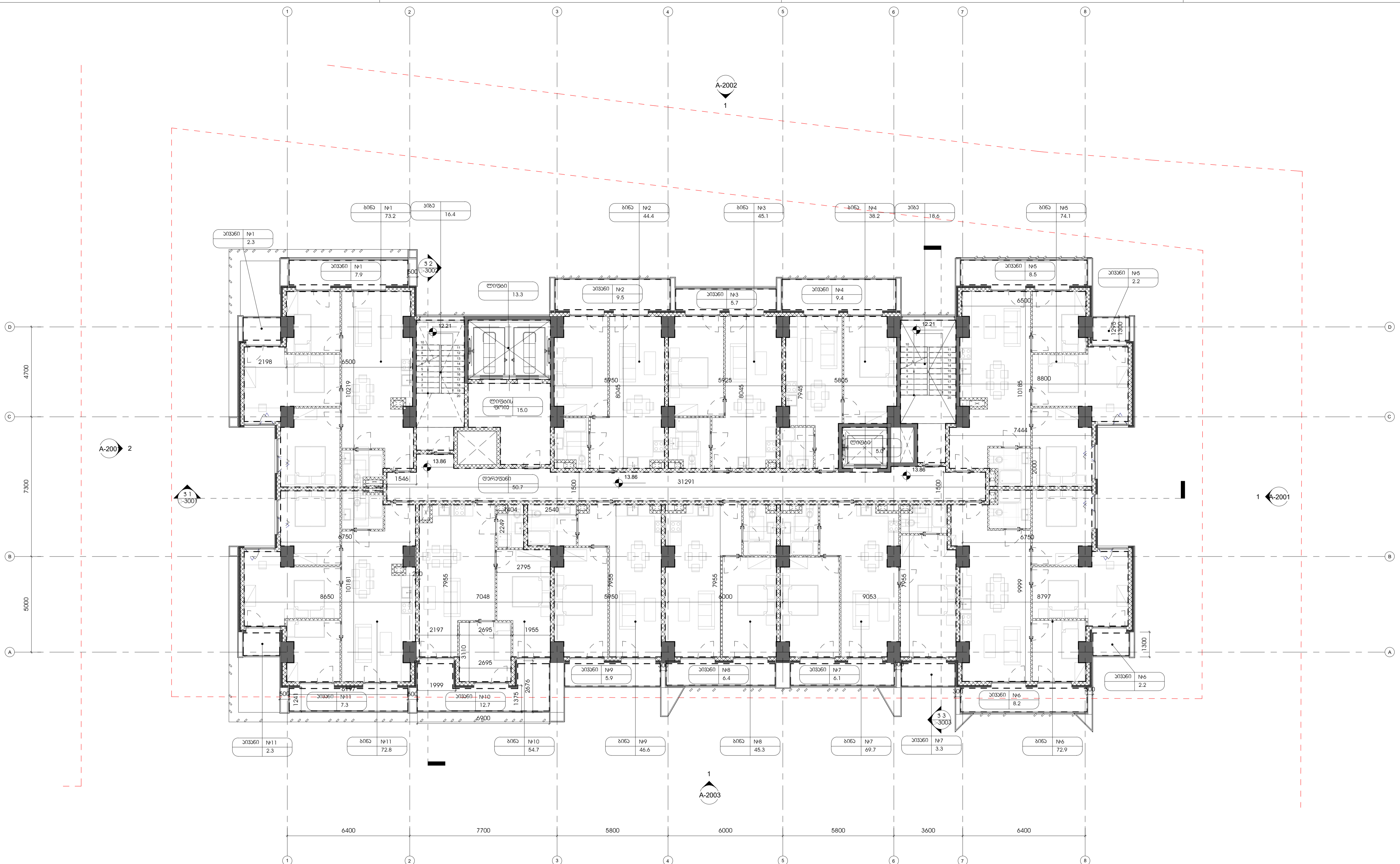
05 1 : 100 ფართობის ცხრილი 5
