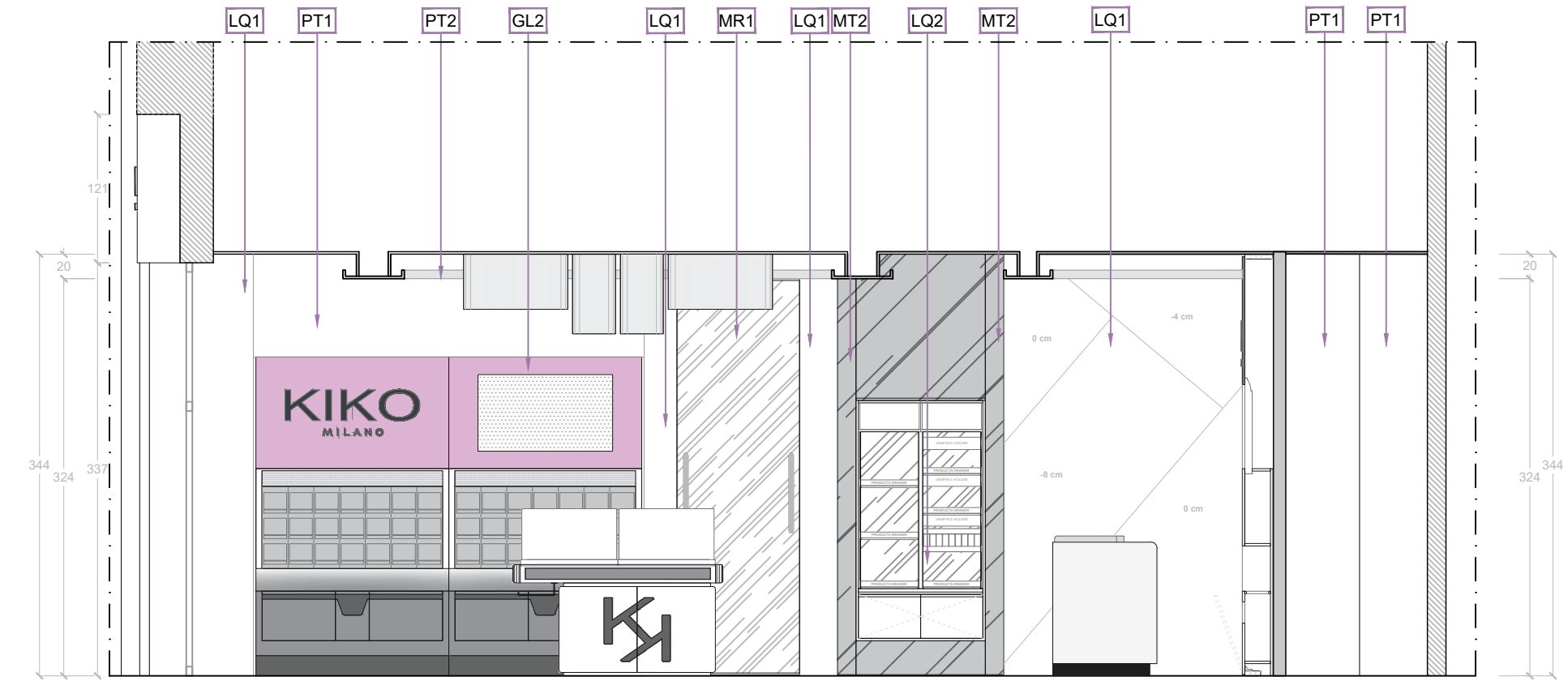
SECTION A-A
